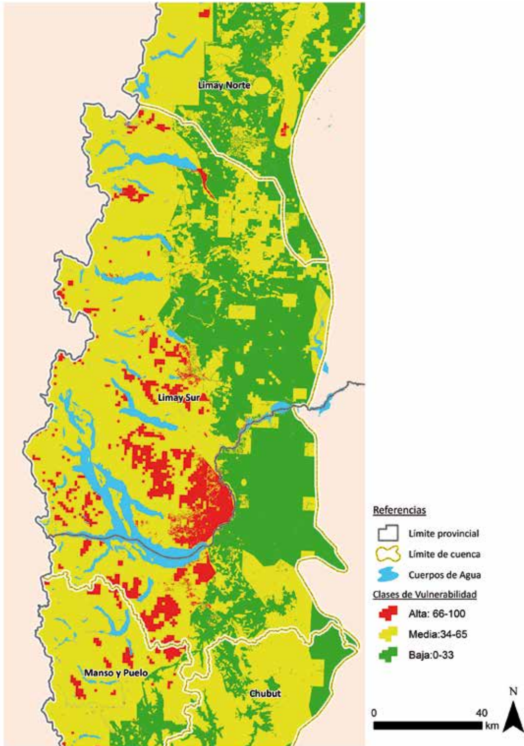
Figura 31. Clases de vulnerabilidad en la cuenca Limay Sur.
